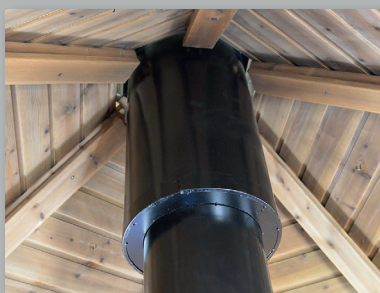
Isoliertes Kaminrohr (Keine Anstände beim Kaminfeger oder Feueraufseher)
