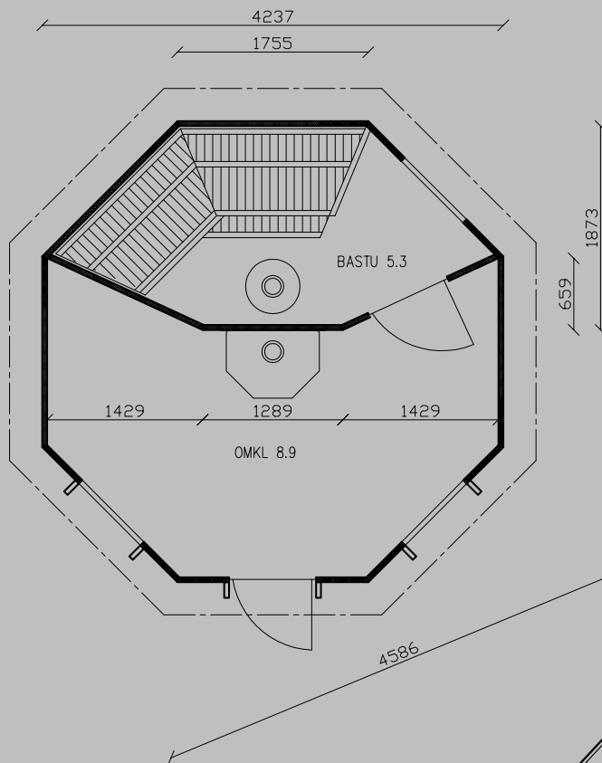
Grundriss
